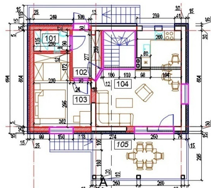
Imamas namo išplanavimas po rekonstrukcijos
