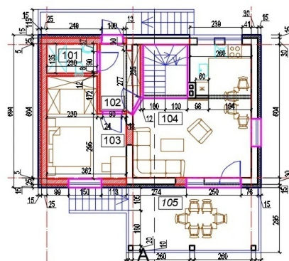
Šalies namo išplanavimas po rekonstrukcijos
