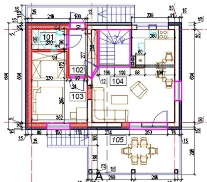
NNTB Pirmas namo išplanavimas po rekonstrukcijos
